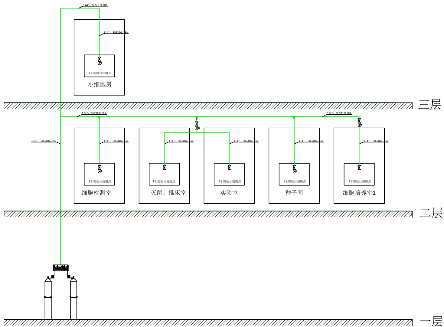
实验室供气系统N2系统图
