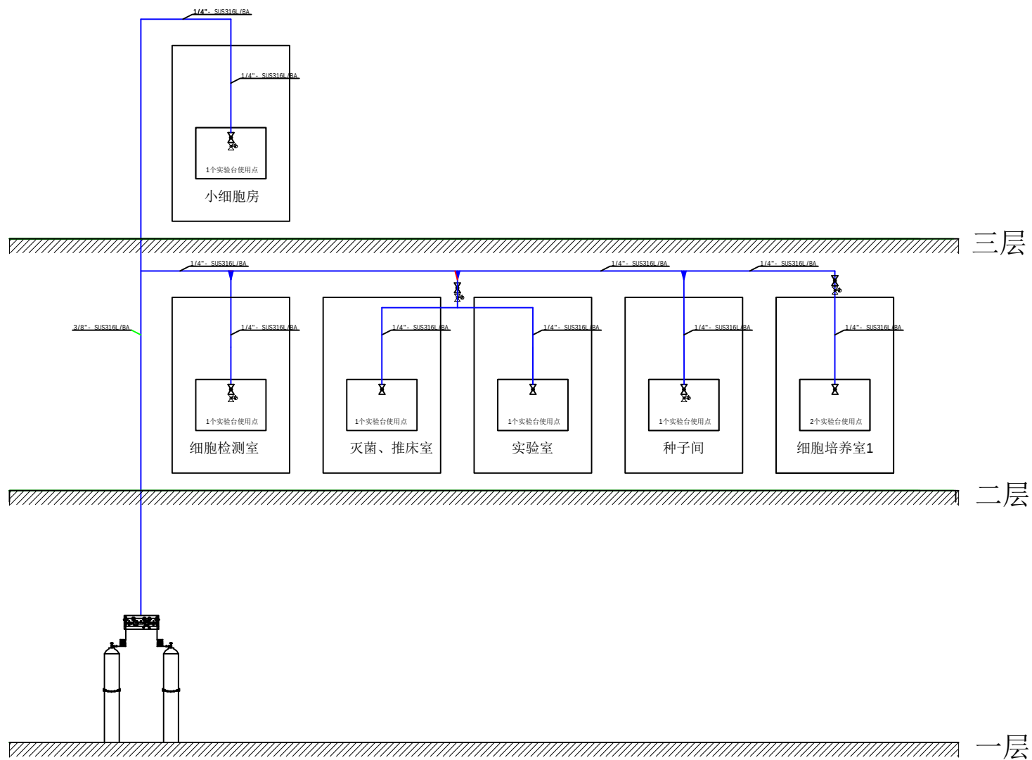
实验室供气系统CO2系统图
