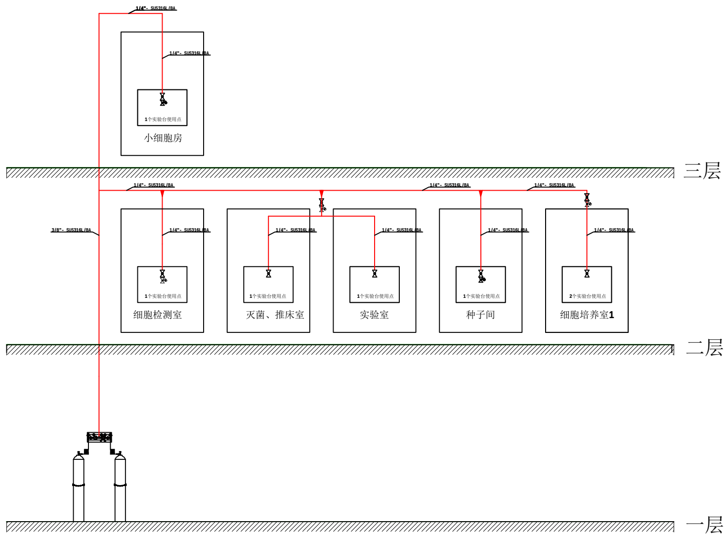
实验室供气系统02系统图
