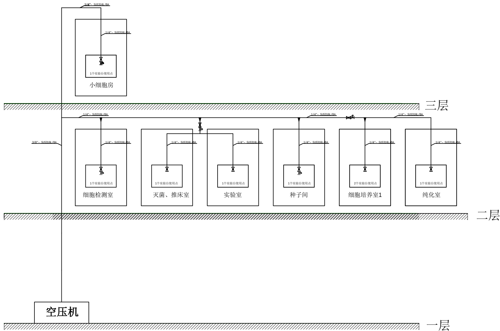
实验室供气系统Air系统图
